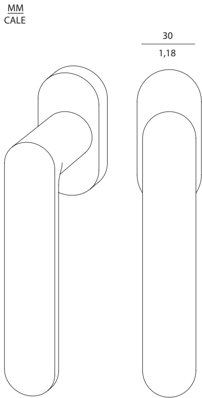
TRZPIEŃ / SPINDLE 7 MM / 0,27 CALA
